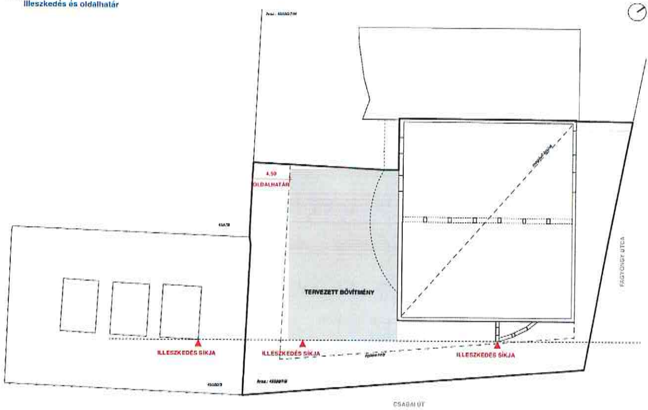
Alaprajz, metszetek, homlokzatok Forrás: beruházói adatszolgáltatás
