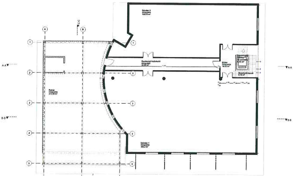
Emeleti alaprajz. Forrás: beruházói adatszolgáltatás
