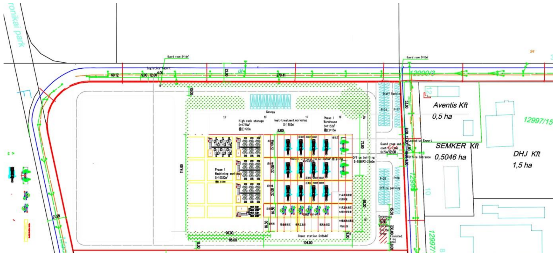
9. ábra: A tervezett létesítmény alaprajzi vázlata
