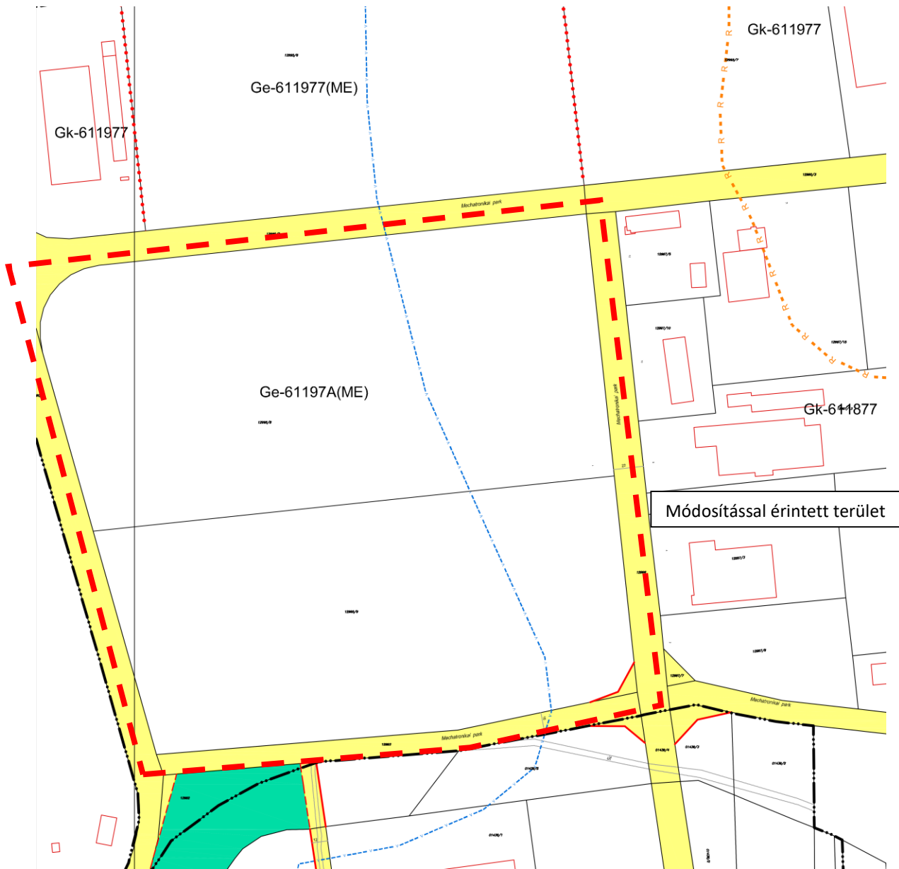
8. ábra: Tervezett szabályozási terv részlet
